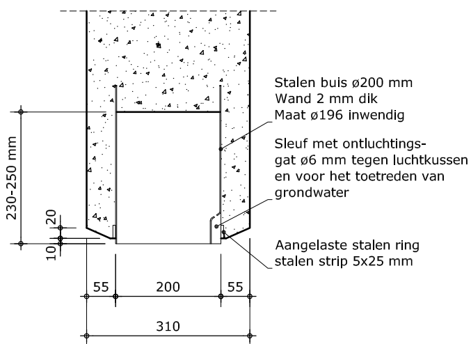
Detail schaal 1:10
